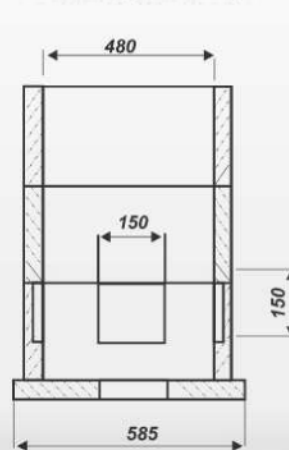
Przekrój poprzeczny
