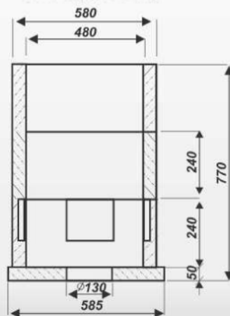
Przekrój podłużny
